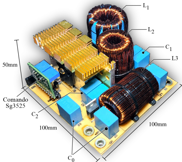
Figura 5. Foto do protótipo do conversor integrado com a célula R^2P^2 e dimensões de 10 cm x 10 cm x 5 cm. Densidade de potência 0,4 W/cm 3 .
