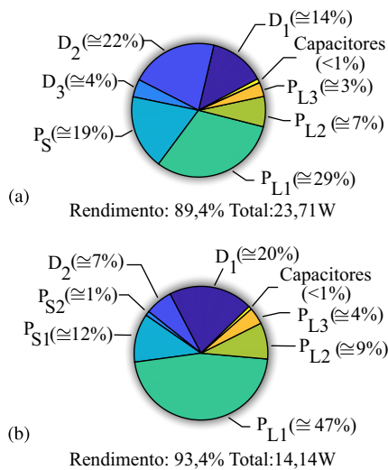
Figura 13. Distribuição teórica das perdas no conversor. Em (a) para o conversor integrado R^2P^2 e (b) para o conversor associado.
