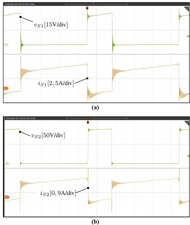
Figura 11. Formas de onda de tensão e corrente nos interruptores do conversor associado. Em (a) no interruptor S_1 e (b) no interruptor S_2 .
