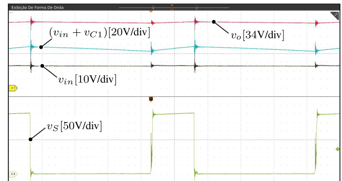
Figura 7. Principais formas de onda de tensão para o conversor integrado com a célula R^2P^2 . Na janela superior são mostradas as formas de onda da tensão de saída v_o , a tensão do primeiro estágio v_b = (v_{in} + v_{C1}) e a tensão de entrada v_{in} . Na janela inferior é mostrada a forma de onda de tensão no interruptor S .
