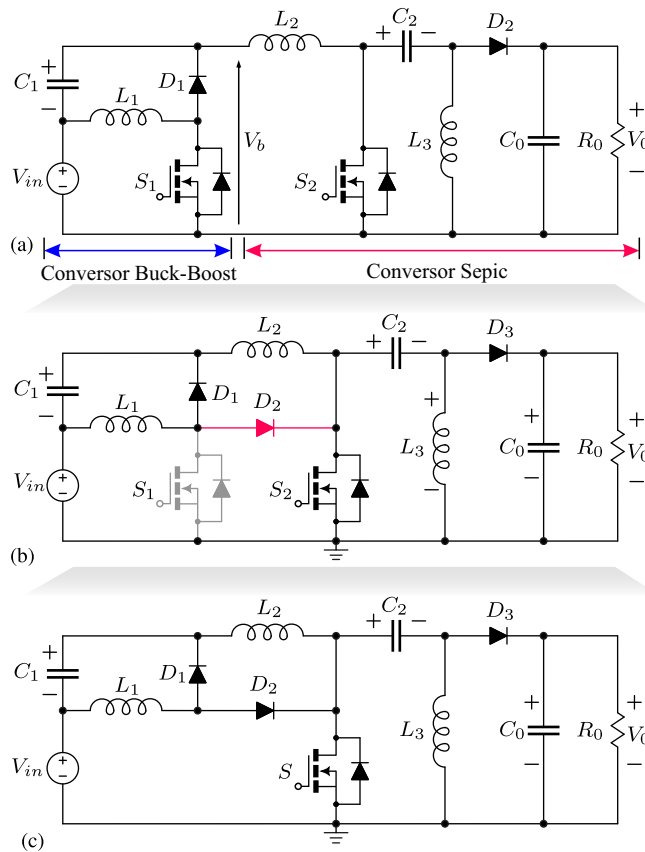
Figura 1. Derivação dos conversores propostos a partir da associação e da integração dos conversores Boost Modificado e SEPIC.
