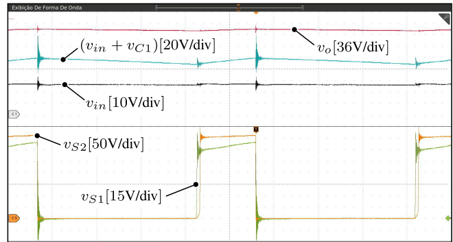
Figura 10. Principais formas de onda de tensão do conversor associado. Na janela superior são mostradas as formas de onda da tensão de saída v_o , a tensão do primeiro estágio v_b = (v_{in} + v_{C1}) e a tensão de entrada v_{in} . Na janela inferior são mostradas as formas de onda de tensão nos interruptores S_1 e S_2 .
