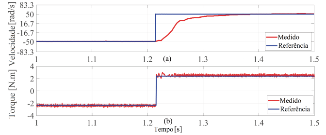
FIGURA 9. (a) Resposta da velocidade e do (b) torque durante o teste de degrau da referência de velocidade - L-FCS-PCC.
