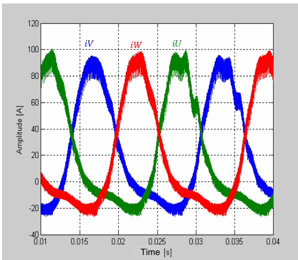
Fig. 14. Input Current
