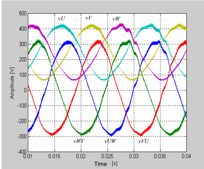
Fig. 13. Output Voltages
