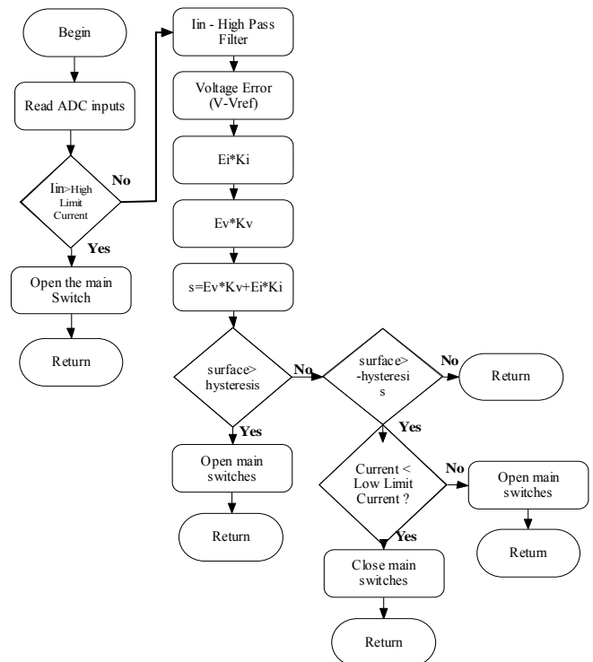
Fig. 12. ADC Interrupt
